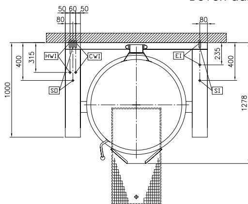
Boven aanzicht
